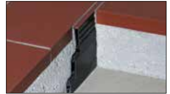
Schlüter-DILEX-MP ist ein Dehnungsfugenprofil mit hinterschnittenen Seitenwänden aus Hart-PVC-Regenerat und einer die Seitenwände überdeckenden Dehnzone aus Weich-Kunststoff mit Verlängerungsprofilen für den Einbau bei Mörtelverlegung. (Produktdatenblatt 4.3)
