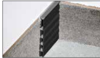
Schlüter-DILEX-EZ 70 ist ein Entspannungs- und Zierprofil mit hinterschnittenen Seitenwänden aus Hart-PVC, mit einer Dehnungszone aus Weich-Kunststoff für den Einbau bei Mörtelverlegung. Die Verlängerungssegmente können entsprechend der Konstruktionshöhe abgetrennt werden. (Produktdatenblatt 4.2)
