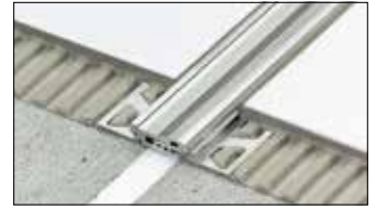
Schlüter-DILEX-BT ist ein Bautrennfugenprofil aus Aluminium mit seitlicher Gelenkanbindung des ineinander verschiebbaren Mittelteils. Somit ist eine dreidimensionale Bewegungsaufnahme möglich. (Produktdatenblatt 4.20)
